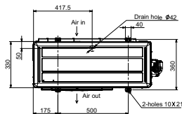
Inwerterowe urządzenia zewnętrzne MUZ, chłodzenie / grzanie MUZ-SF50VE
