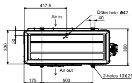
Inwerterowe urządzenia zewnętrzne MUZ, chłodzenie / grzanie MUZ-GF60-71VE
