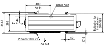
Inwerterowe urządzenia zewnętrzne MUZ, chłodzenie / grzanie MUZ-FH25-35VE
